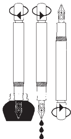
Füllhalter mit Kolbenmechanik
